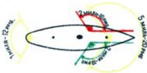
План расположения ходовых огней
