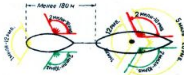
План расположения огней на буксирующем и буксируемых судах
