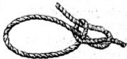
Беседочный узел
