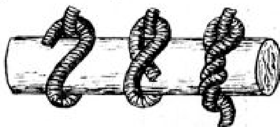
Удавка
