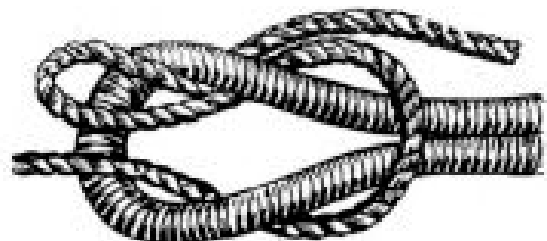
Рифовый узел
