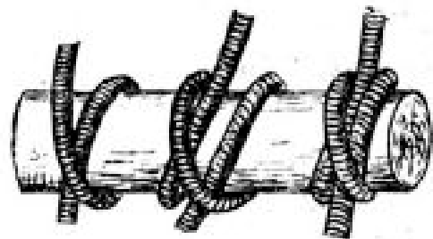
Выбленочный узел
