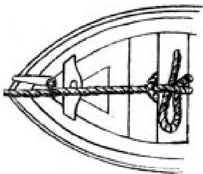
Шляпачный узел
